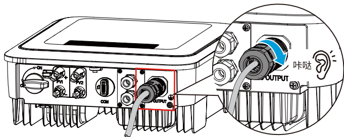
交流连接器-1
